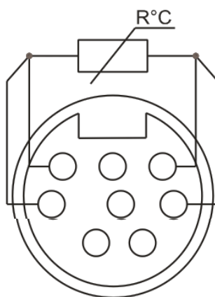
Рисунок 7.2 Входной преобразователь – термпреобразователь сопротивления
